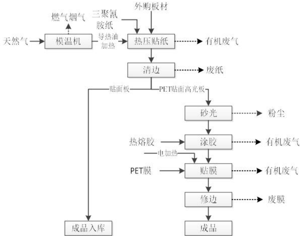
图 2-1 贴面板、PET 贴面高光板生产工艺流程及产污环节示意图
